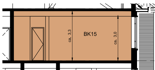
Doorsnede
